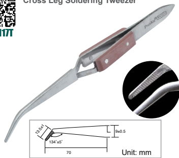
Cross Leg Soldering Tweezer
