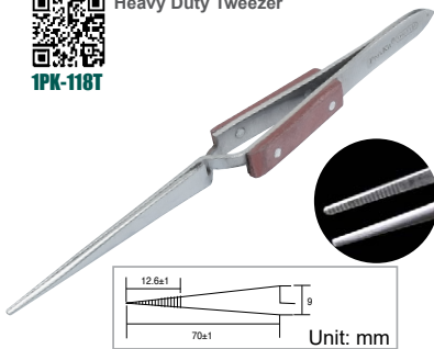
Heavy Duty Tweezer
